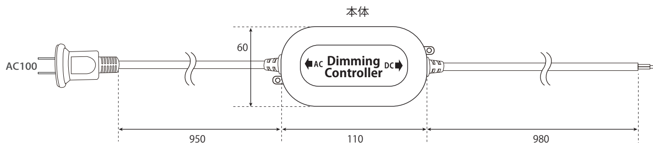
正面図
