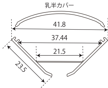
端面図
