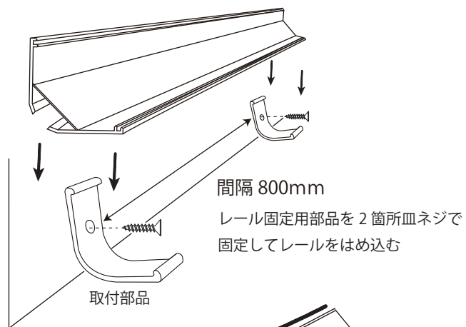
取付方法
