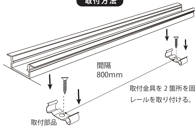
取付方法
