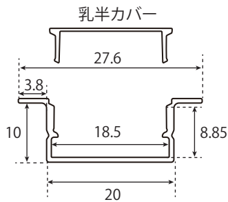
本体取付図
