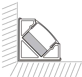
本体取付図
