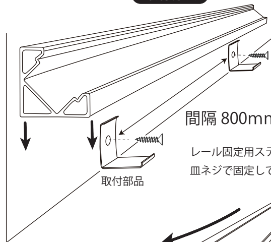
取付方法
