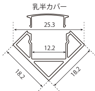
端面図
