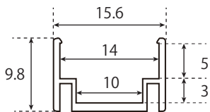
端面図
