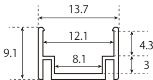
端面図
