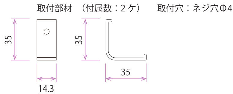
全体図
