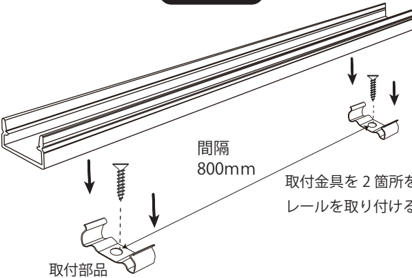
取付方法
