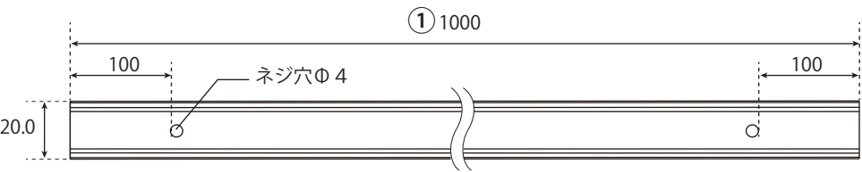
正面図
