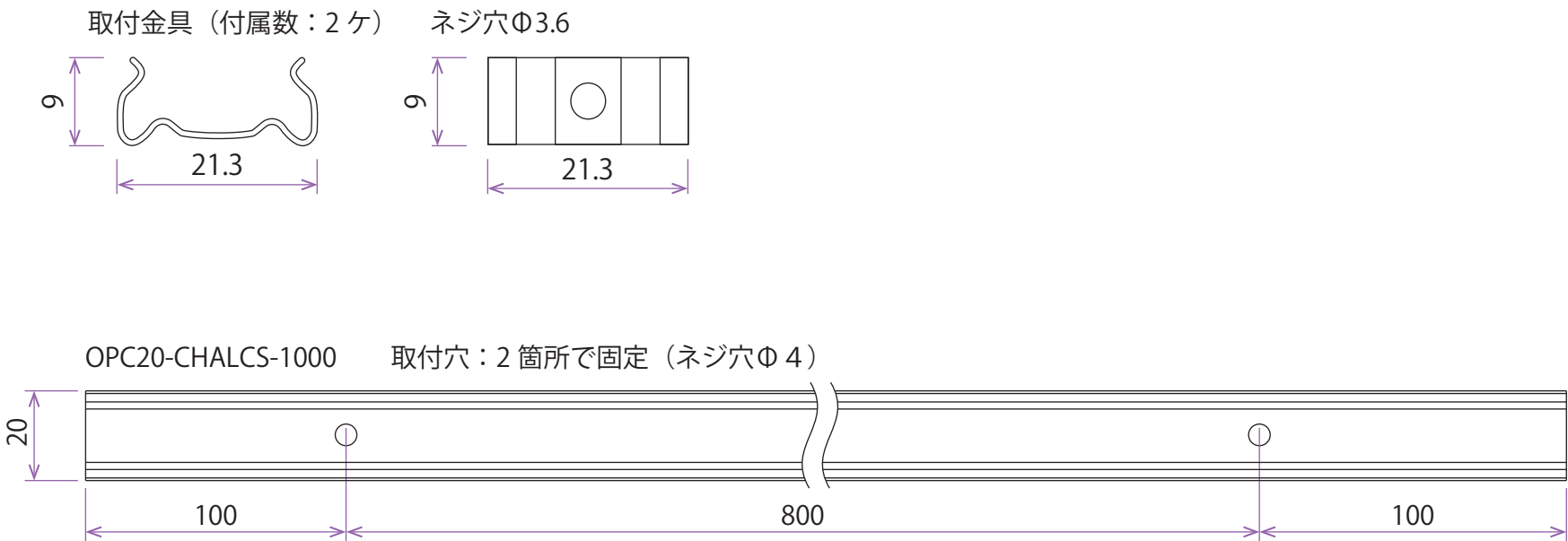
全体図
